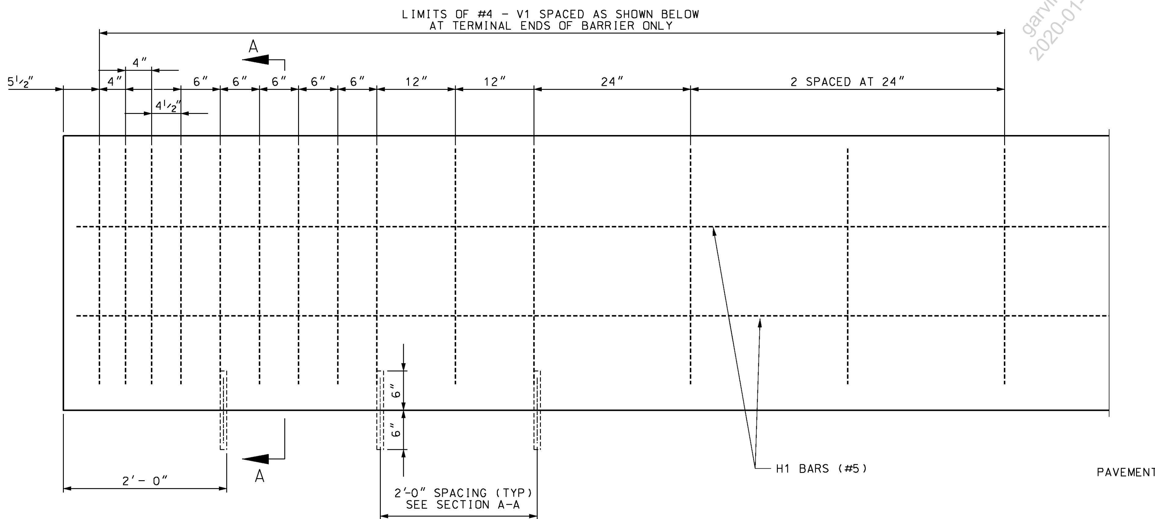
ELEVATION
